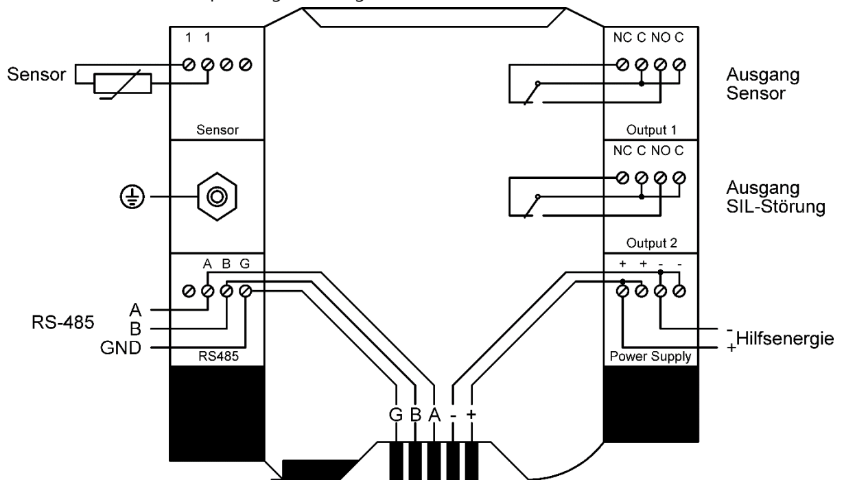
Abbildung III.c: Verdrahtungsplan
