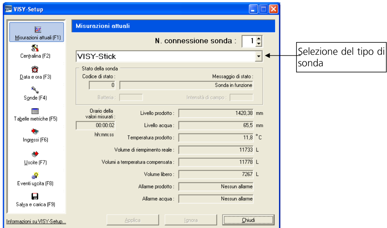
Figura 4: Esempio di valori di misurazione attuali (configurati)
