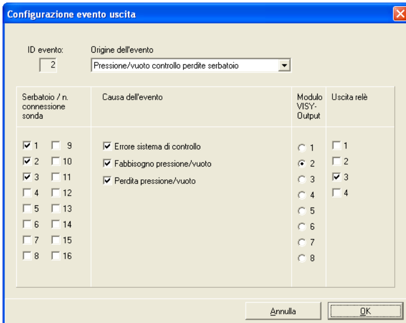
Figura 29: Editor eventi uscita
