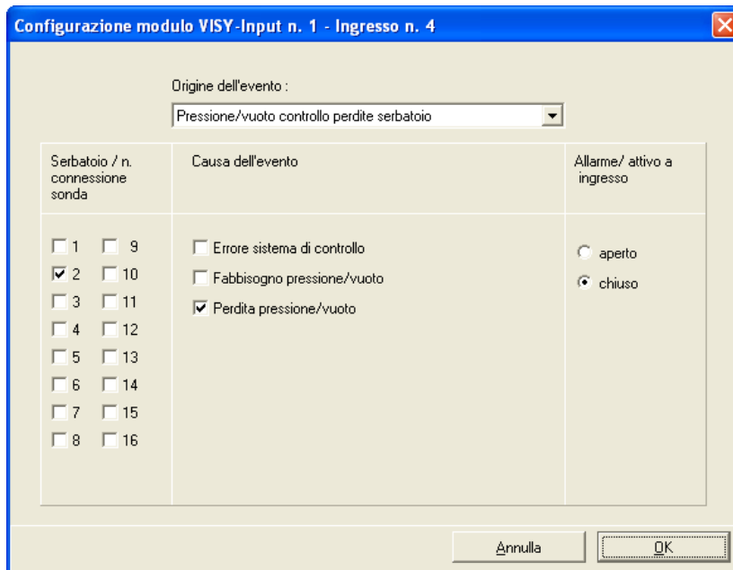
Figura 26: Editor eventi ingresso, per la configurazione di un singolo ingresso
