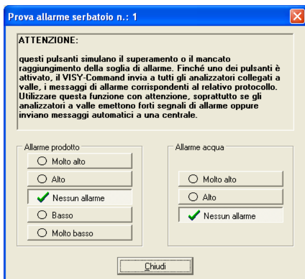
Figura 20: Finestra di test dei sei allarmi
