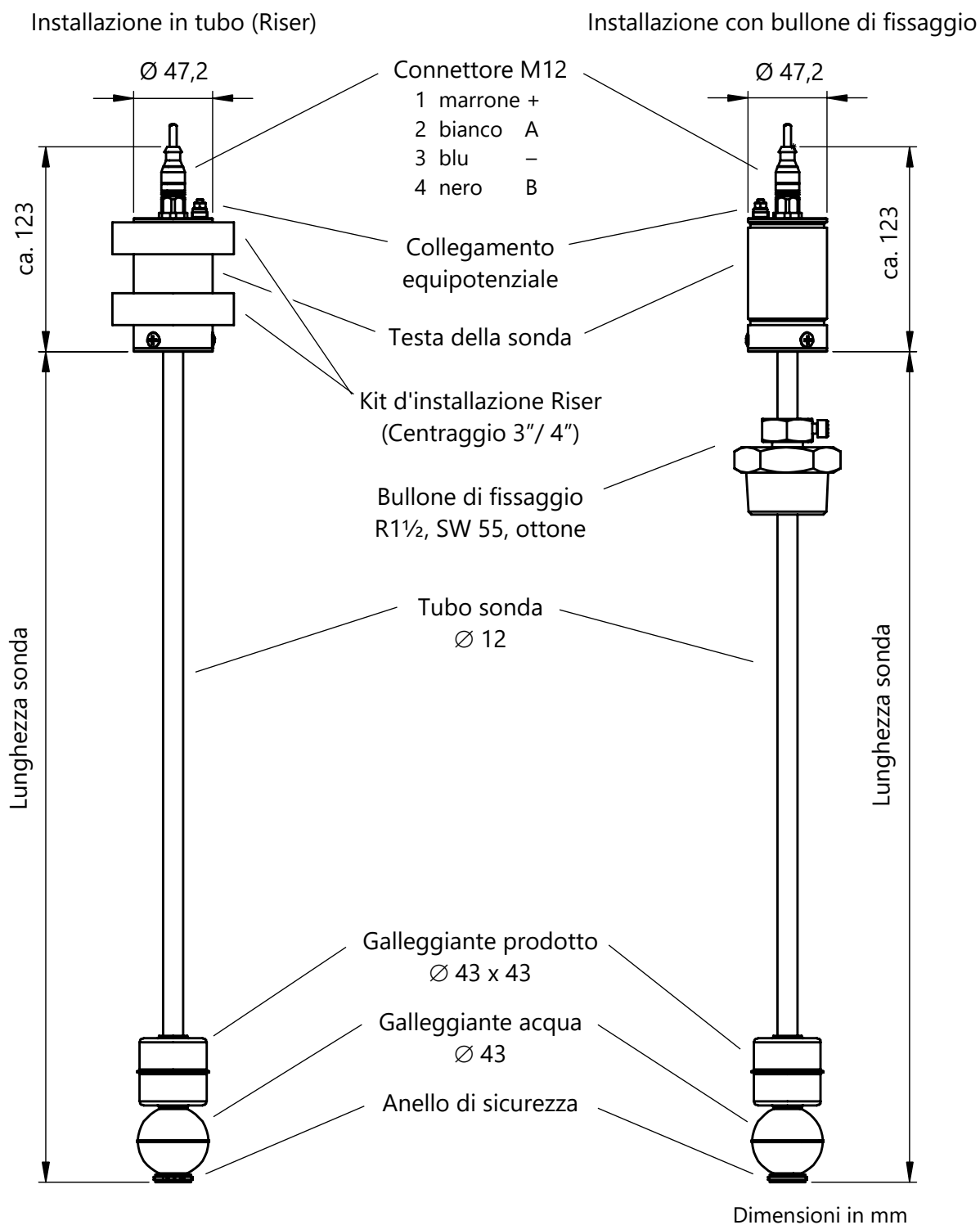
Figura 2: VISY-Stick / Biodiesel / E15
