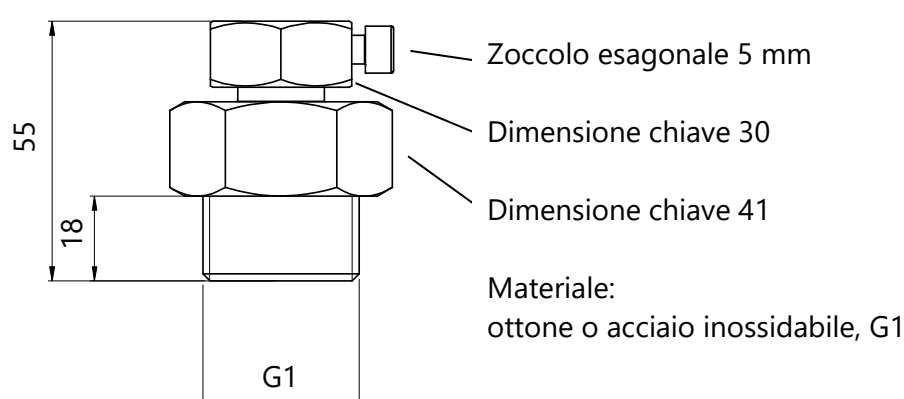
Figura 20: Bullone di fissaggio da 1"
