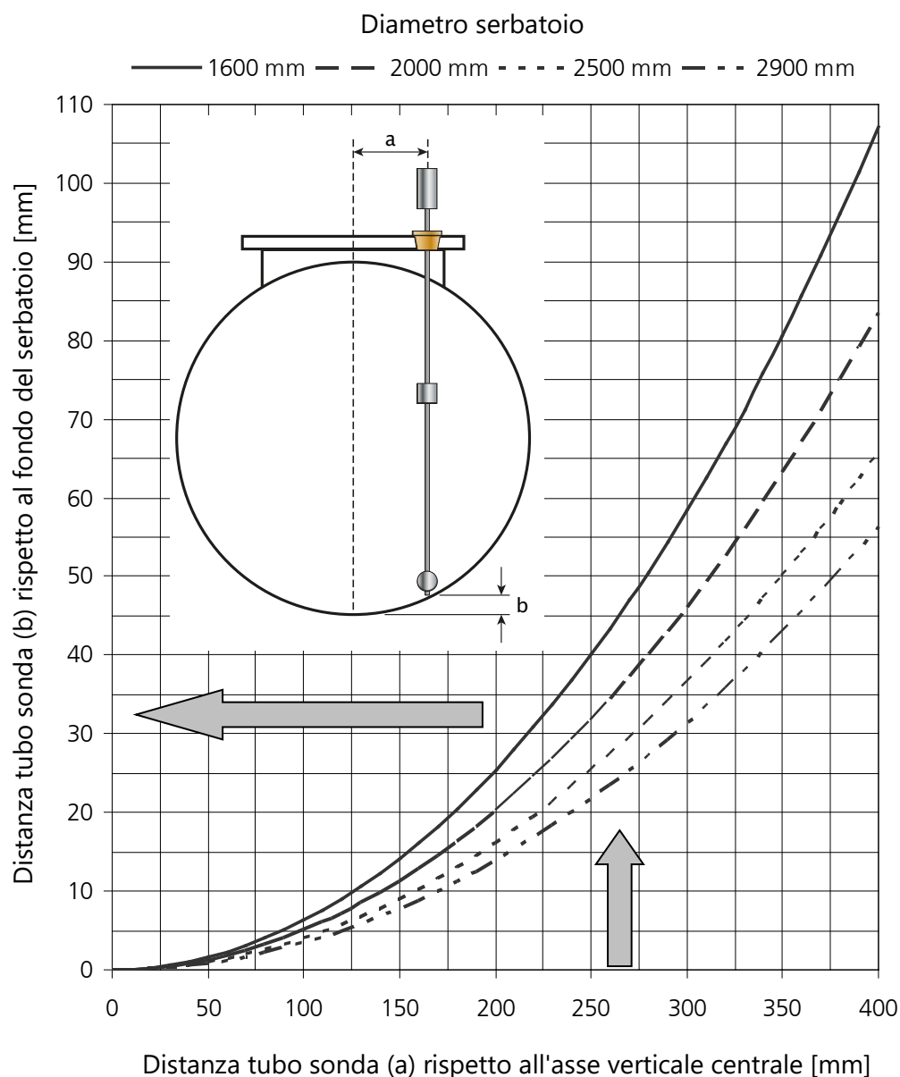
Figura 22: Offset d'installazione
