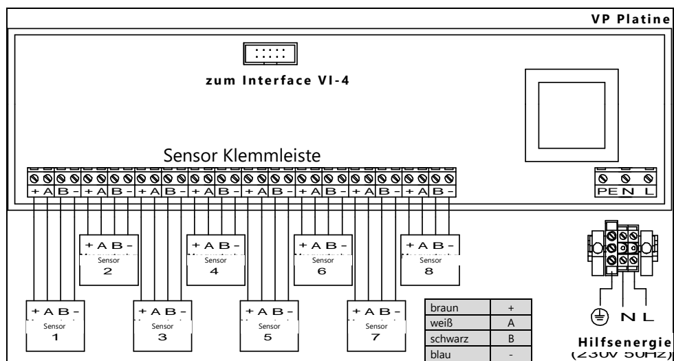
Abbildung 1: VISY-Command 8 mit einer VP-1 Platine für 8 Sensoren
