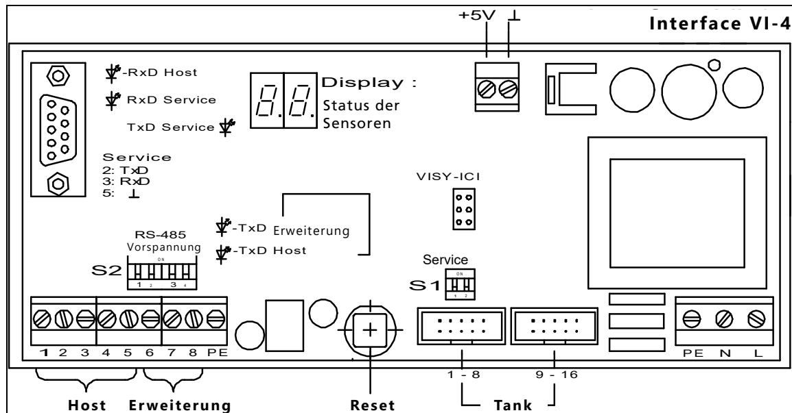
Abbildung 3: VI-4 Interface
