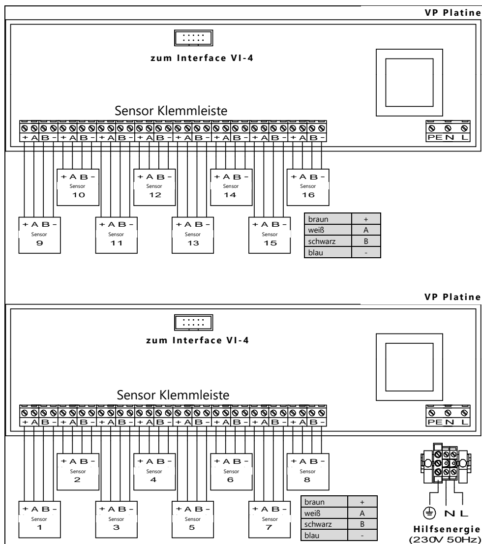
Abbildung 2: VISY-Command 16 mit zwei VP-1 Platinen für 16 Sensoren
