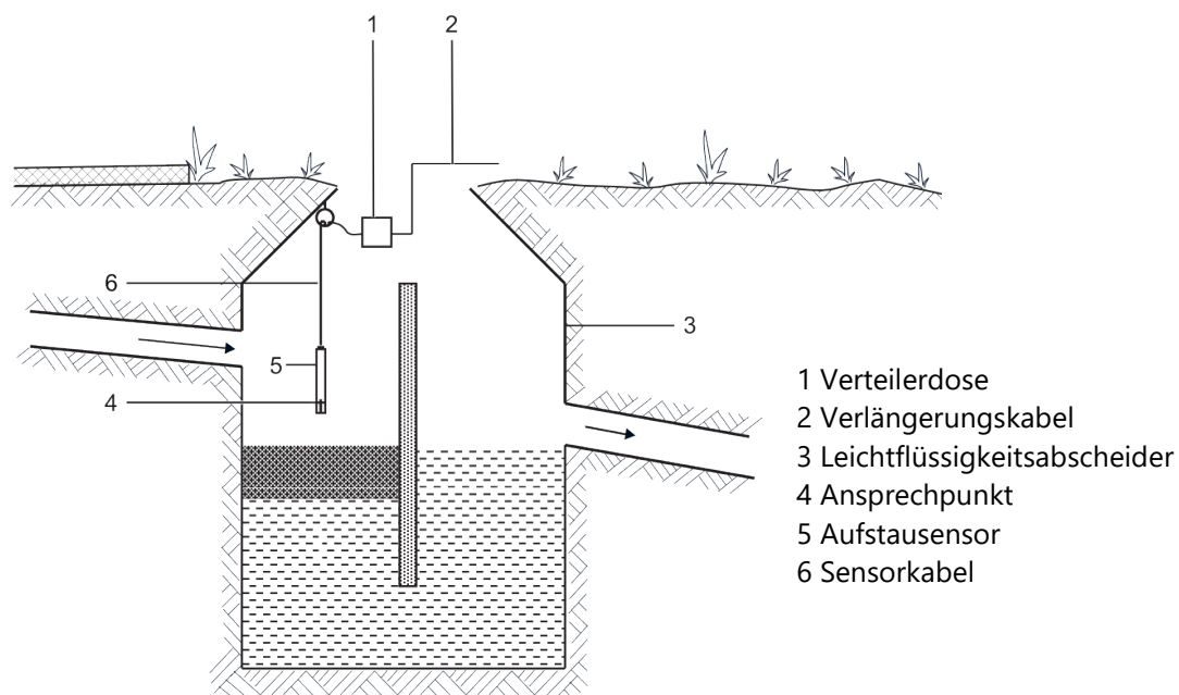
Abbildung 4: SEPARIX-T, Installation
