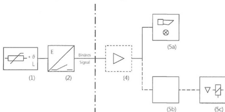
Schematische Darstellung der Überfüllsicherung
