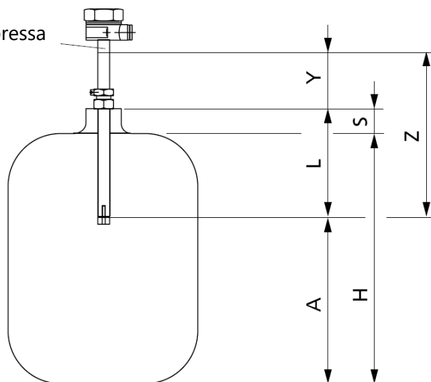
Figura 6: Istruzioni di regolazione
