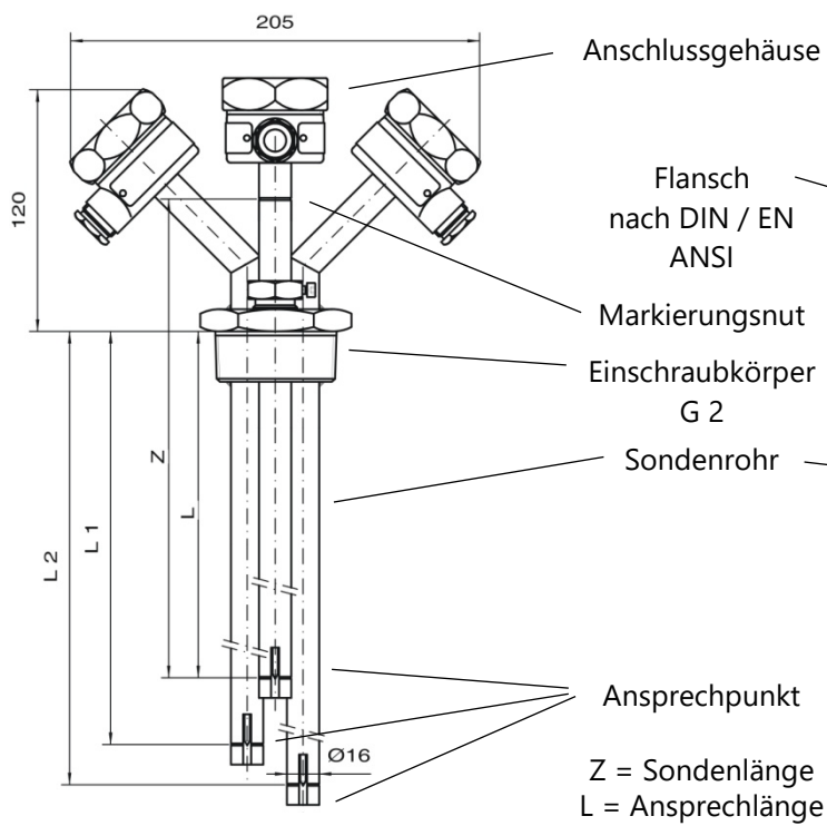
Abbildung 11: 76 A Trio 3
