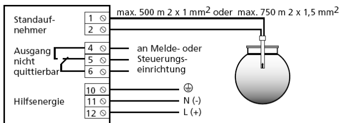
Abbildung 16: Anschlusschema NB 220 H
