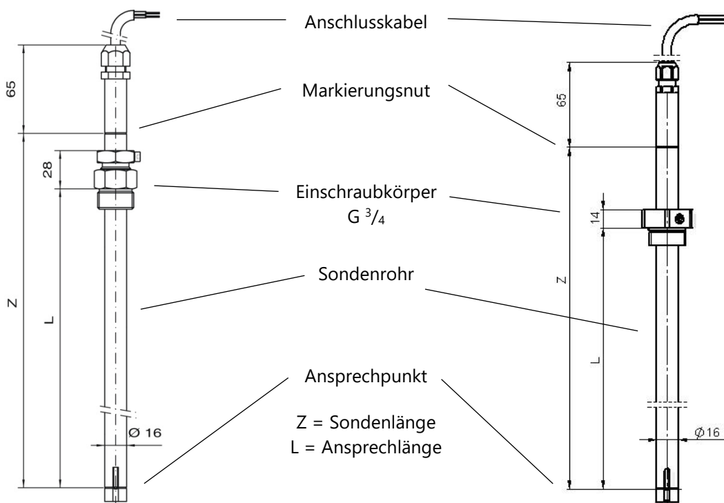
Abbildung 3: 76 C
