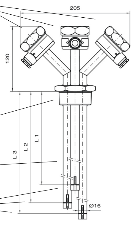
Abbildung 10: 76 A Trio 1
