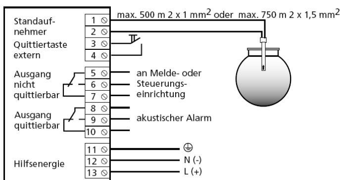
Abbildung 18: Anschlusschema NB 220 QSF
