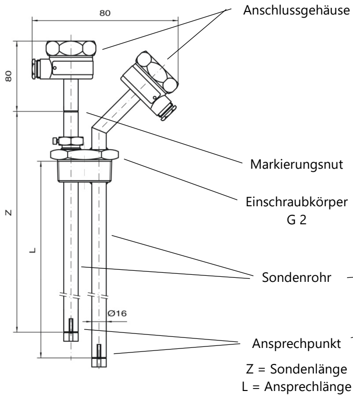
Abbildung 9: 76 A Duo 3
