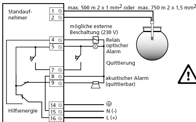
Abbildung 17: Anschlusschema NB 220 QS
