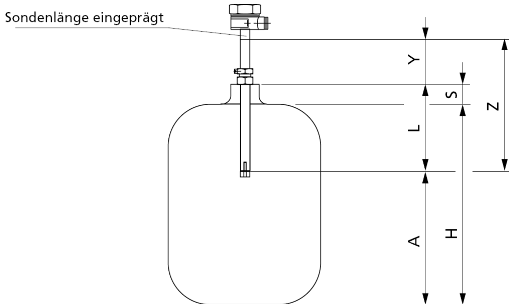
Abbildung 19: Einstellhinweise
