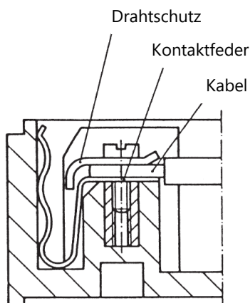
Abbildung 22: Kabelmontage
