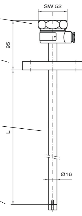
Abbildung 12: 76 A F
