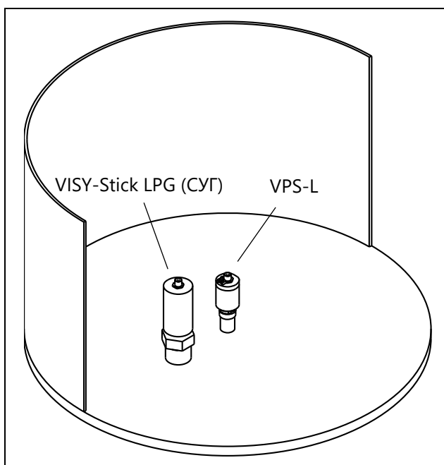
Рисунок 3: Монтаж в крышке резервуара
