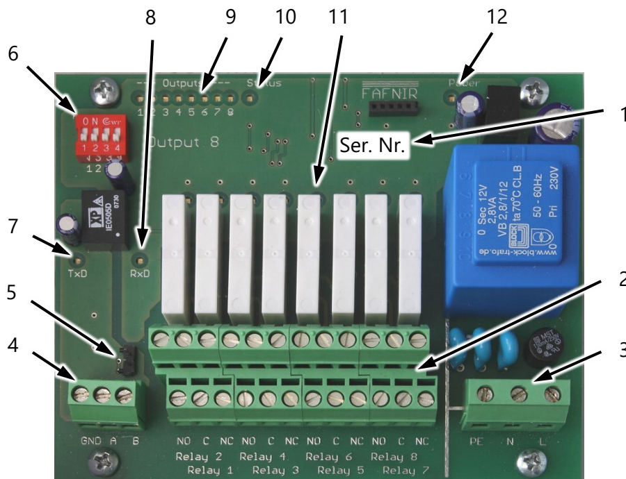
Abbildung 1: Aufbau VISY-Output 8
