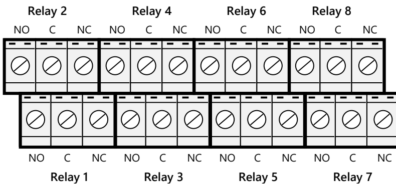
Abbildung 3: Schraubklemme Relaiskontakte
