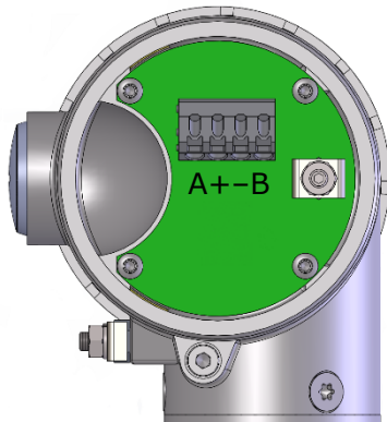
Figura 11: Compartimiento de conexión TORRIX (Ex) XTS
