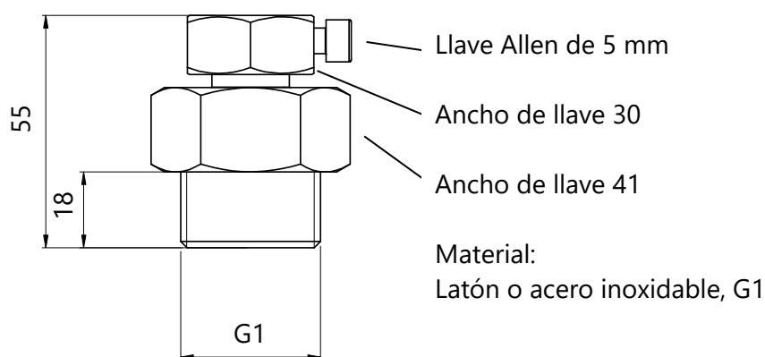
Figura 18: Unidad a rosca de 1"
