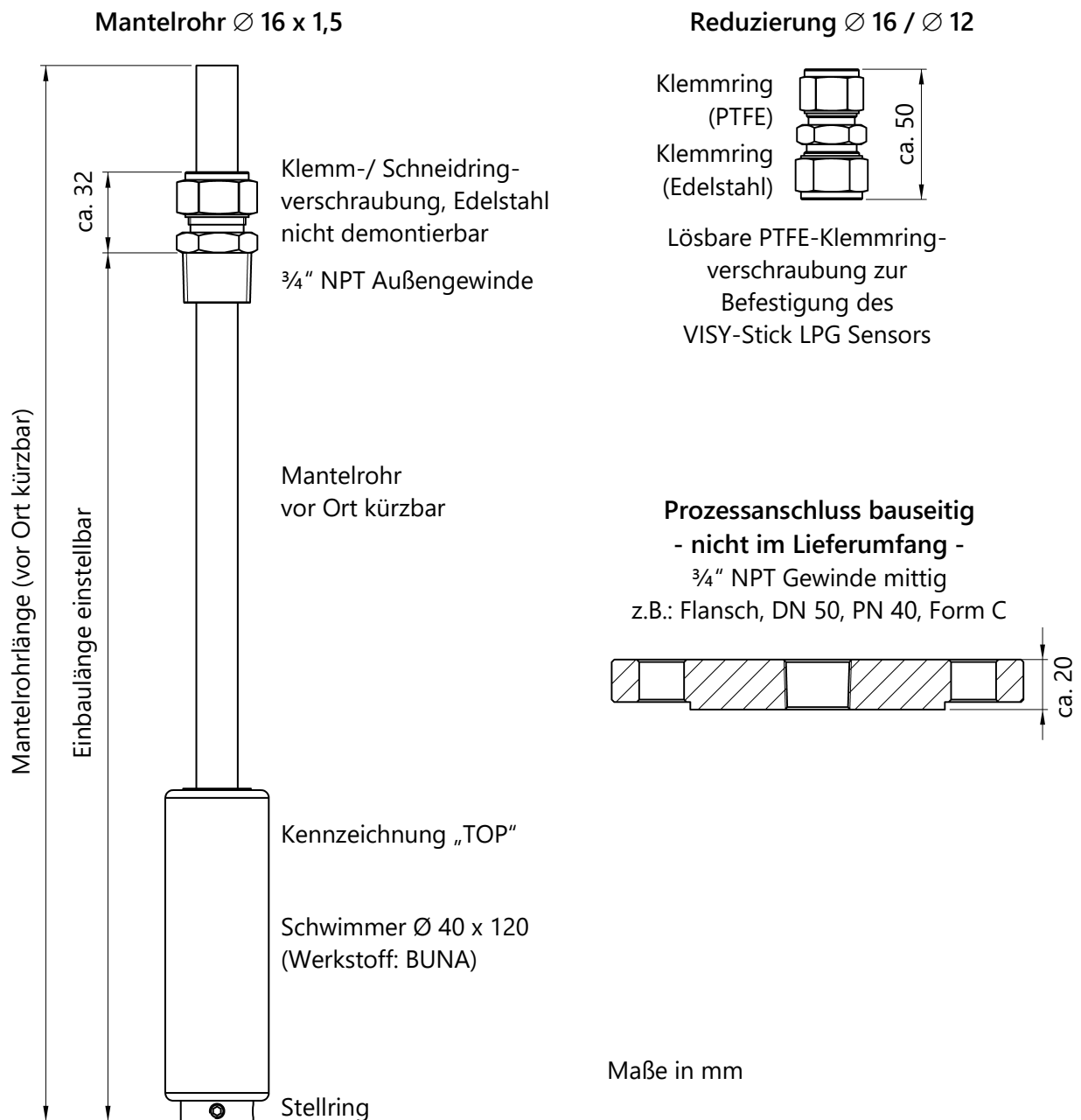
Abbildung 17: Variables LPG-Einbaukit für Flüssiggasbehälter
