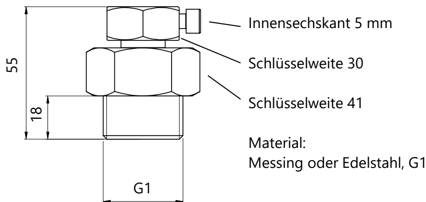
Abbildung 18: 1" Einschraubkörper
