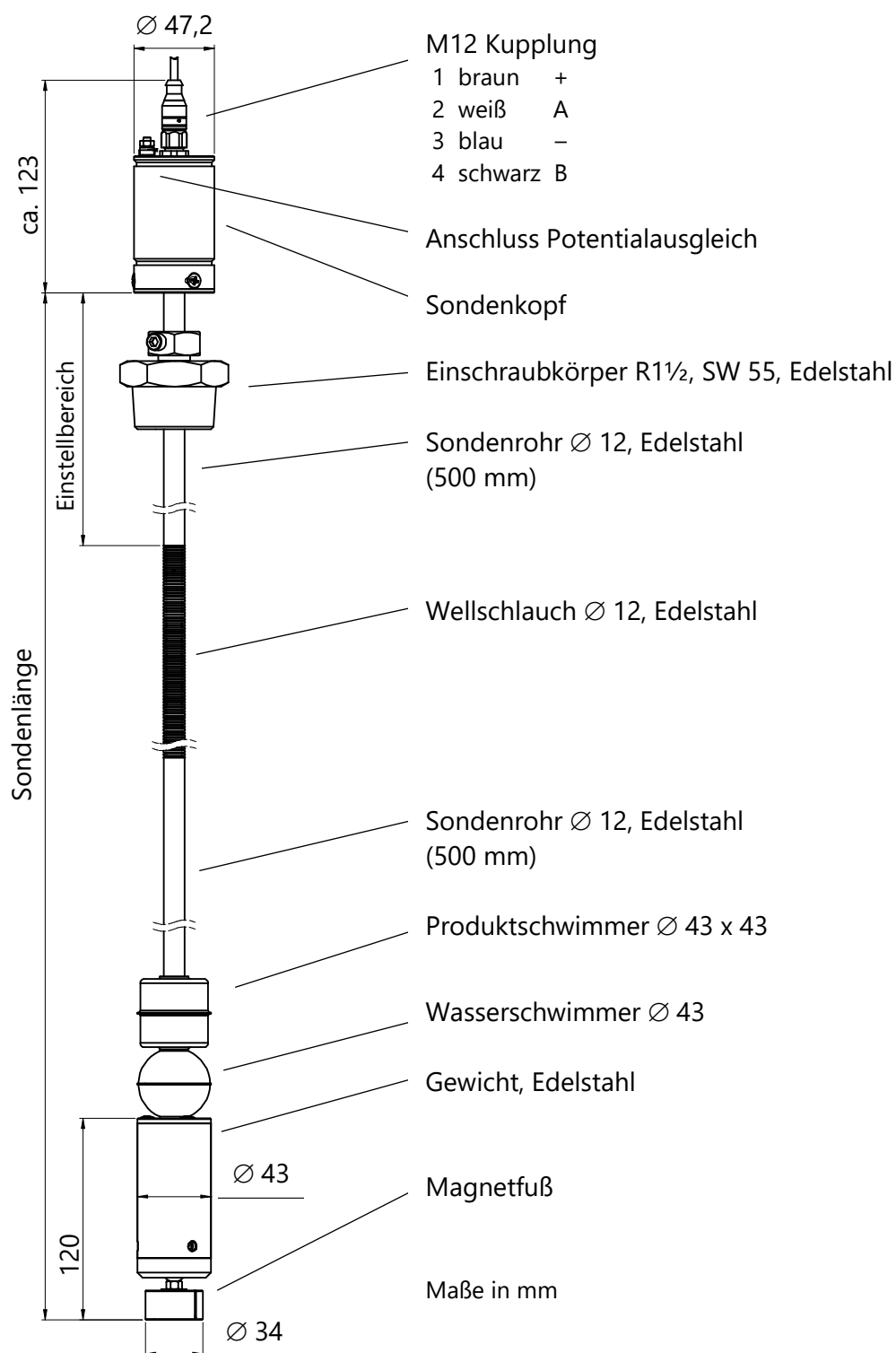
Abbildung 7: VISY-Stick Flex
