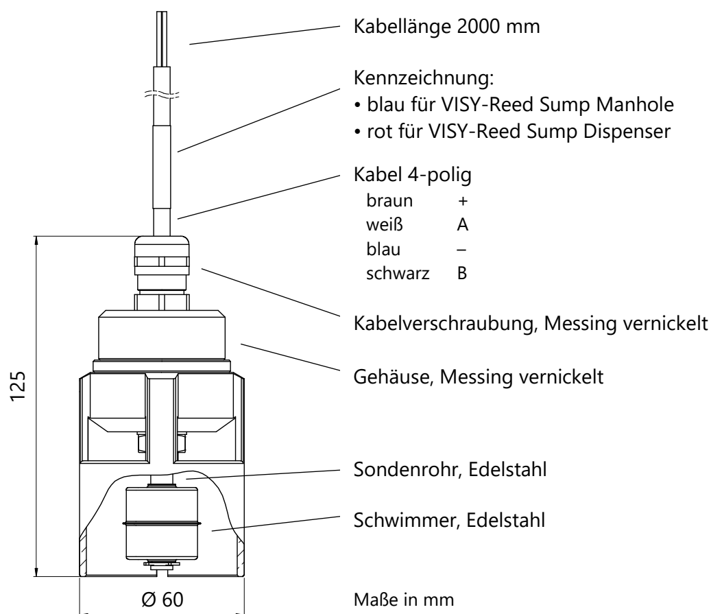
Abbildung 12: VISY-Reed Sump
