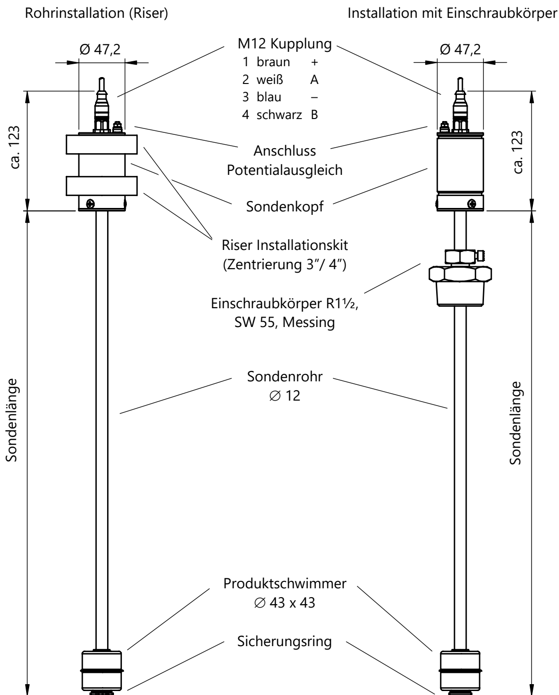
Abbildung 4: VISY-Stick Ethanol
