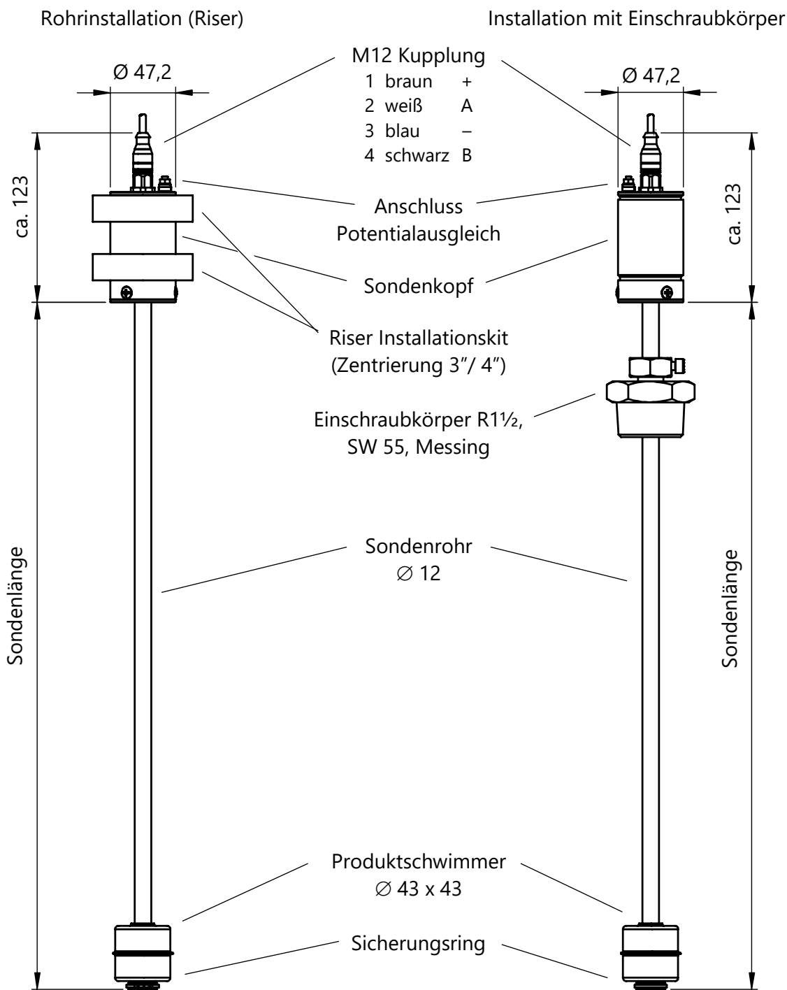
Abbildung 9: VISY-Stick Interstitial
