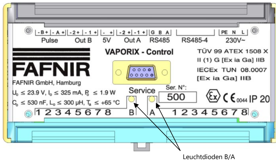
Abbildung 6: VAPORIX-Control LEDs
