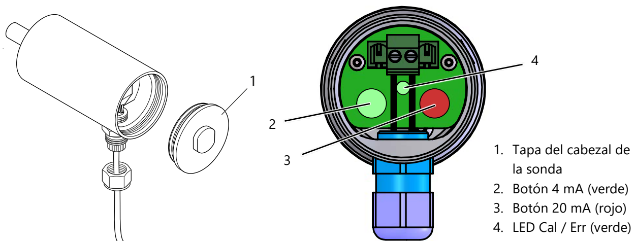
Figura 11: Carcasa de conexión del cabezal de la sonda
