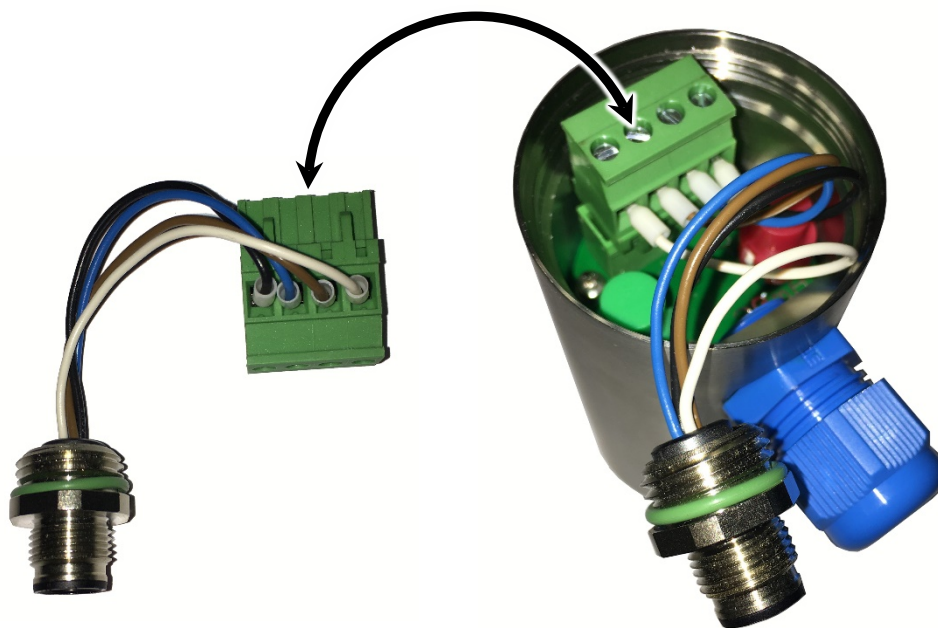
Figura 12: Conexión del adaptador M12
