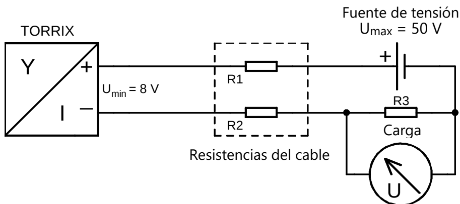
Figura 7: Esquema de conexión TORRIX
