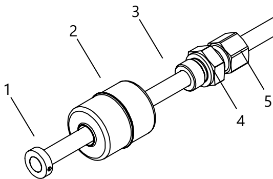
Figura 4: Montaje con unidad a rosca
