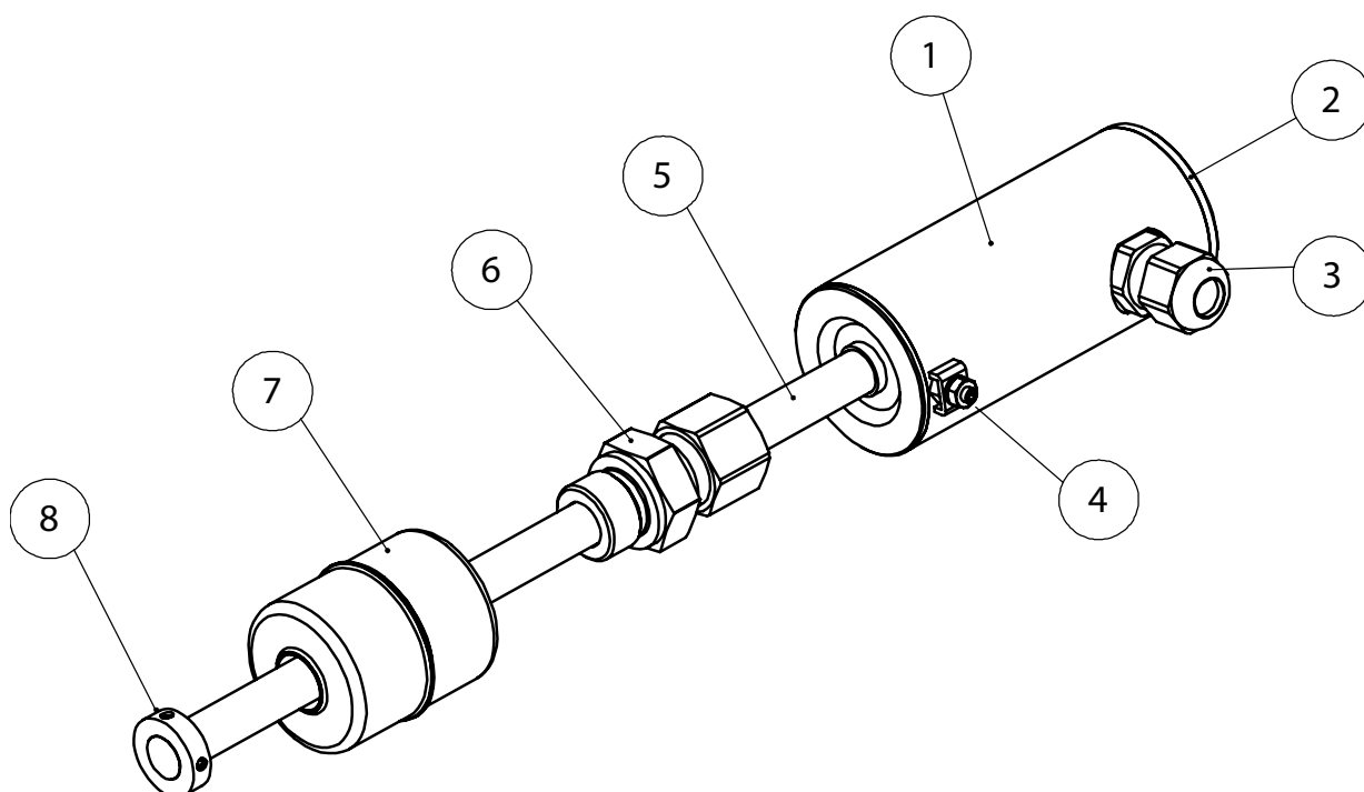
Figura 1: Sensor del nivel de llenado TORRIX 5.5
