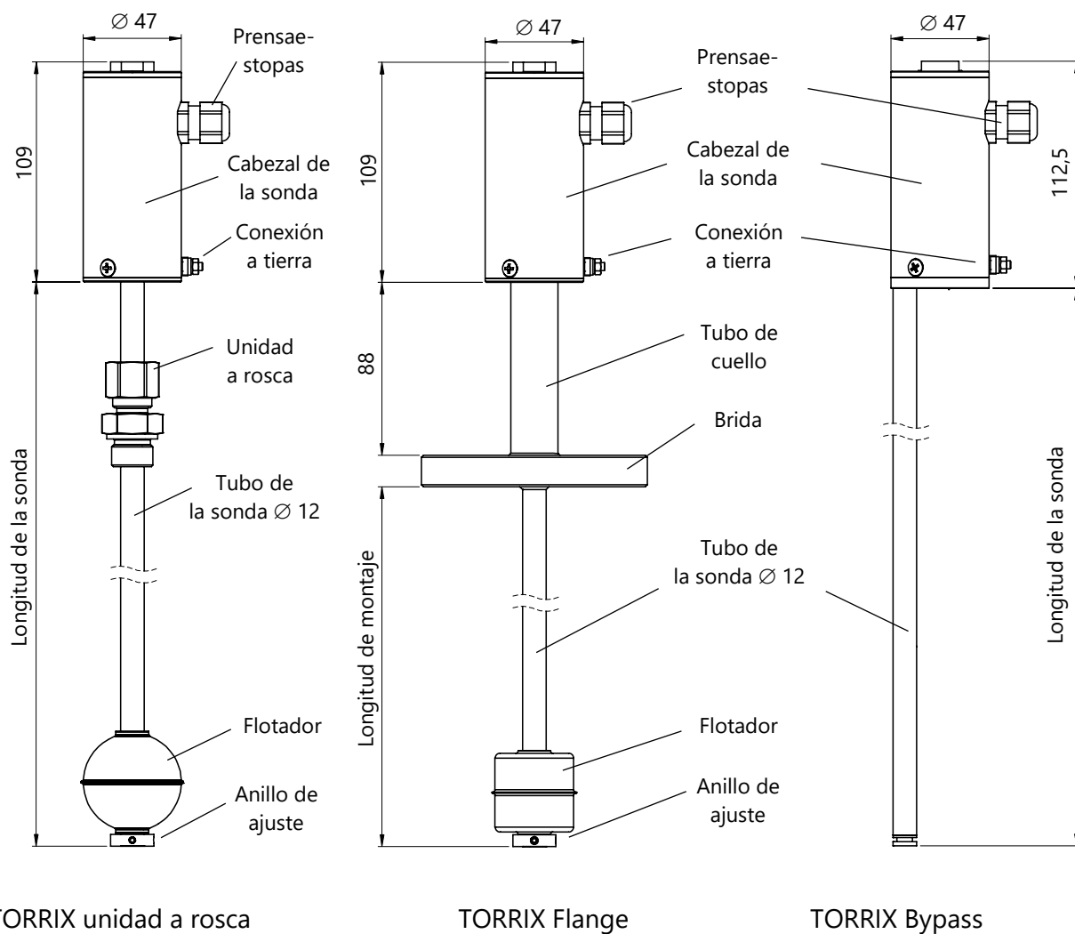
Figura 3: Versiones de TORRIX
