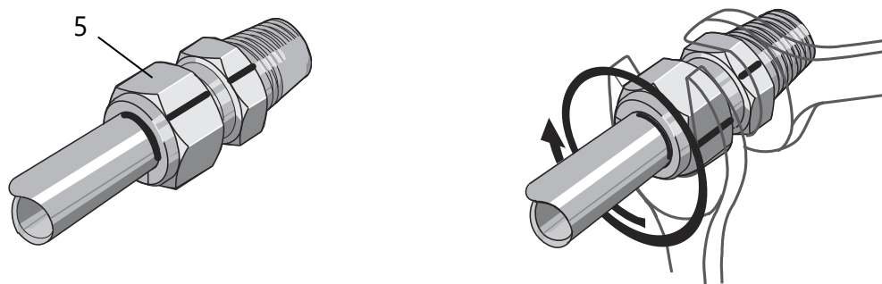
Figura 5: Fijación del racor de compresión
