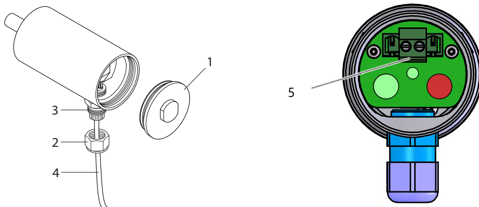
Figura 9: Cableado
