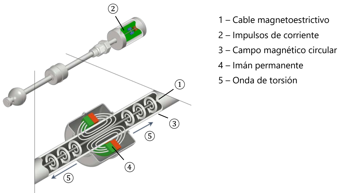
Figura 2: Principio de funcionamiento del sensor de nivel de llenado TORRIX
