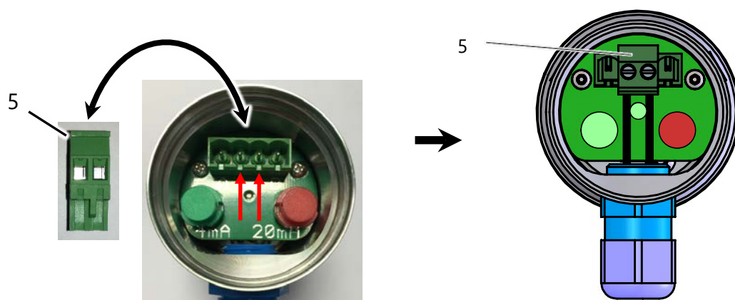
Figura 10: Terminal de tornillos extraíble
