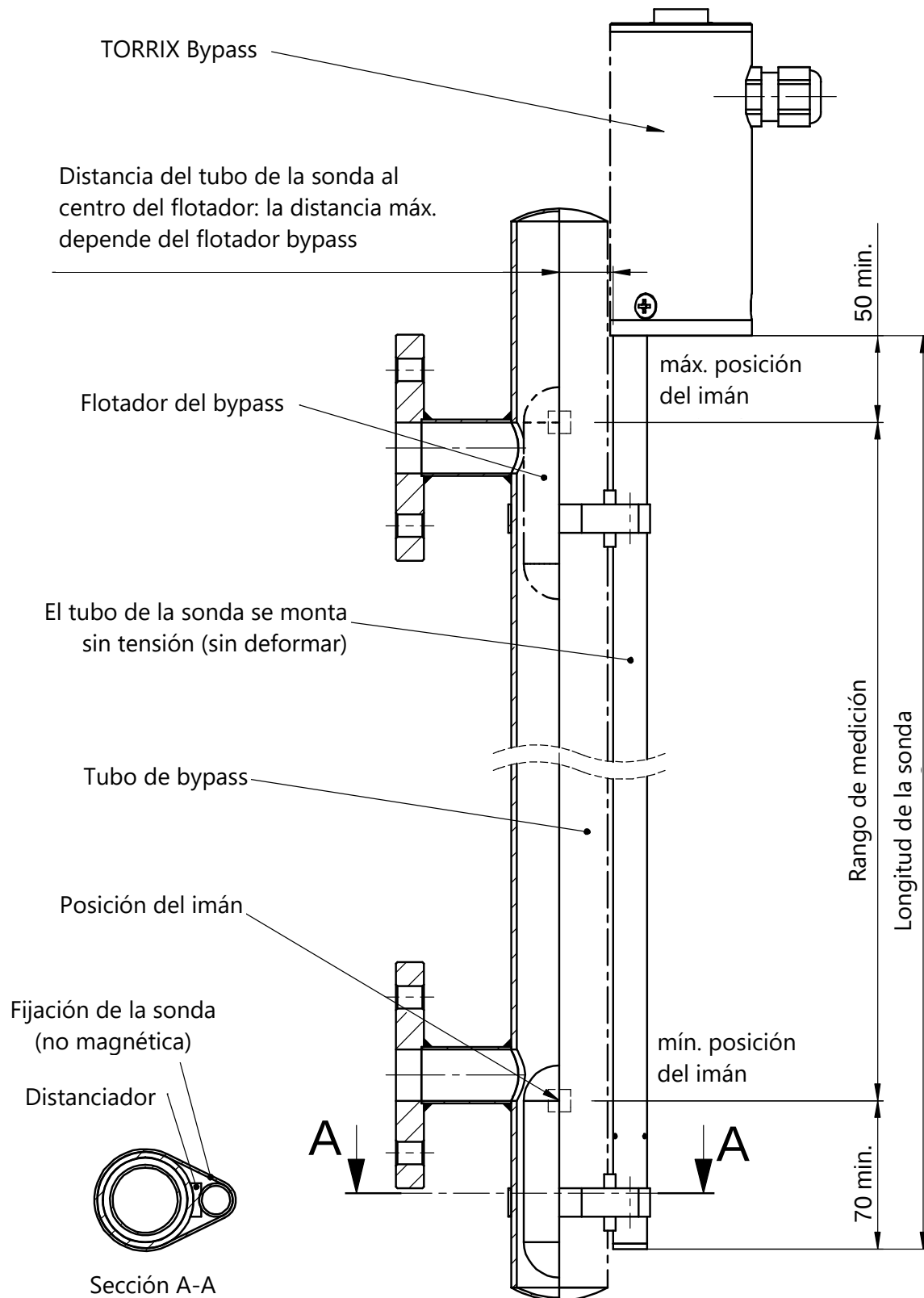
Figura 6: Instalación con Bypass
