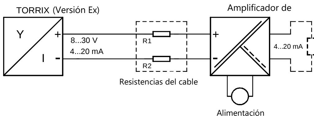
Figura 8: Esquema de conexión TORRIX Ex
