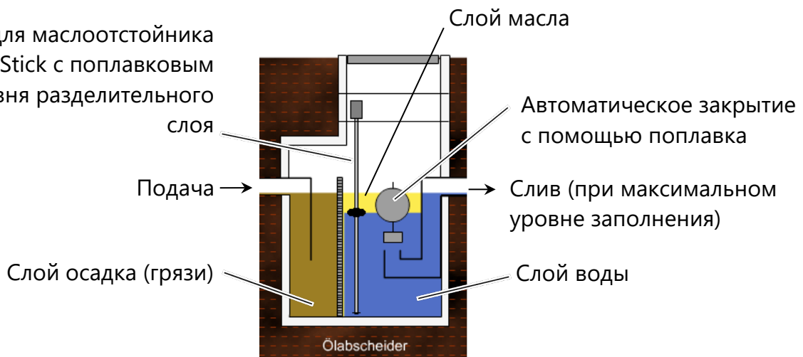
Рис. 14: Масляный сепаратор с зондом масляного сепаратора VISY-Stick
