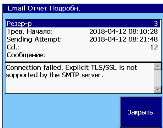
Рис. 17: Электронный отчет
