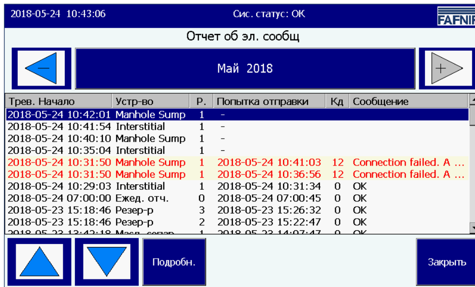
Рис. 17: Электронный отчет
