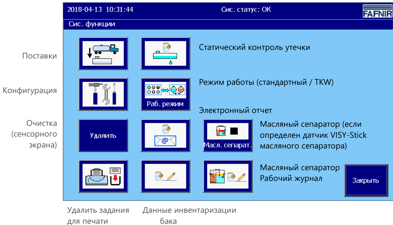
Рис. 5: Системные функции
