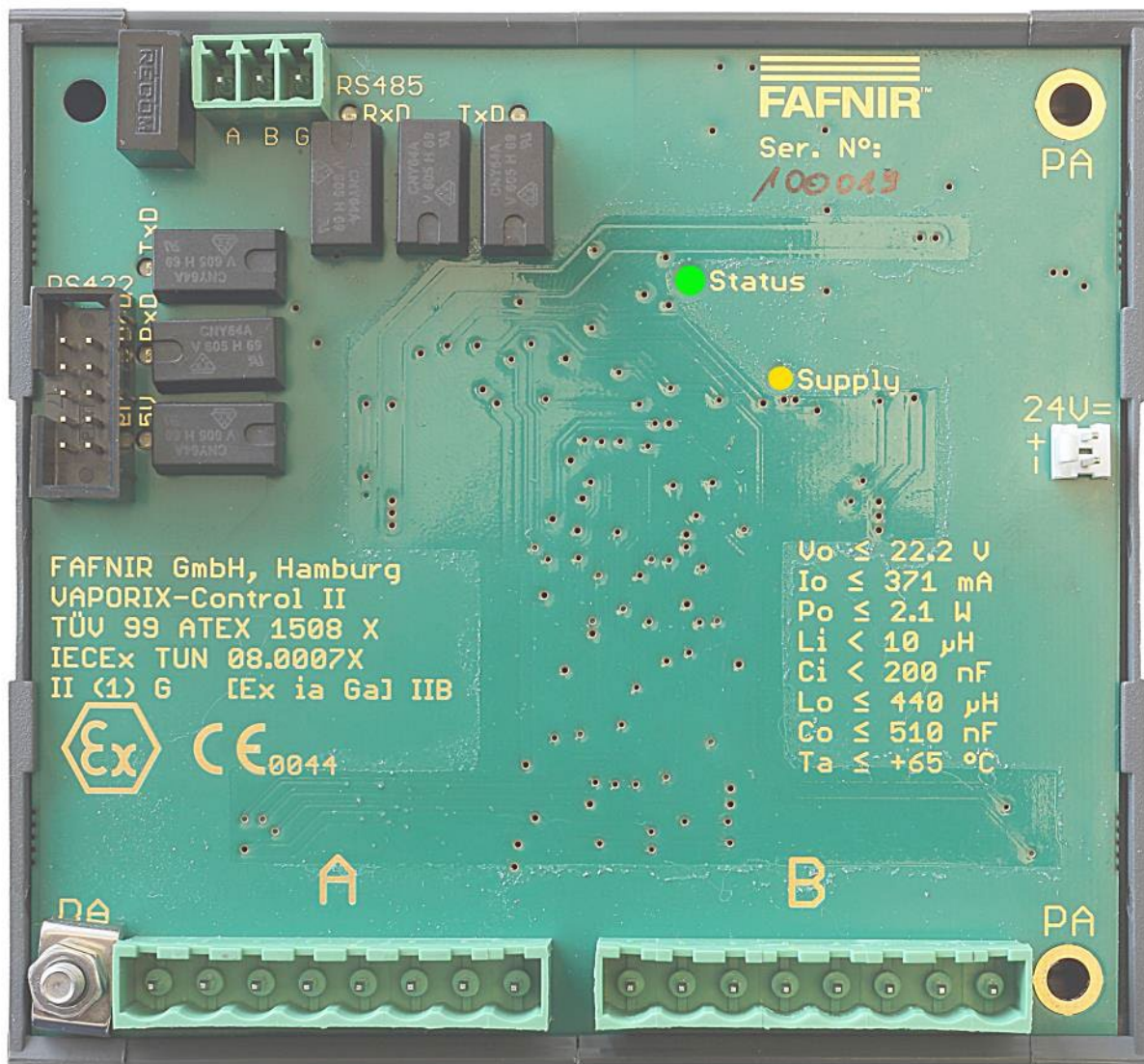
Image 5 : Unité d'analyse VAPORIX-Control II
