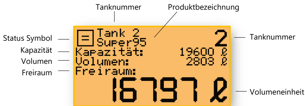
Abbildung 1: Beispiel für die Anzeige der Tankdaten
