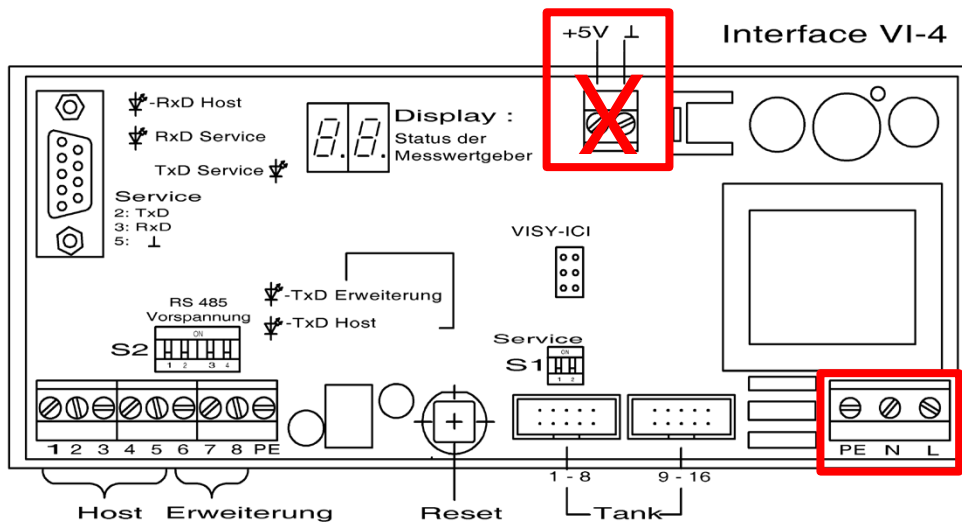
Abbildung 3: Klemmen N und L der Versorgungsspannung des Interface VI-4
