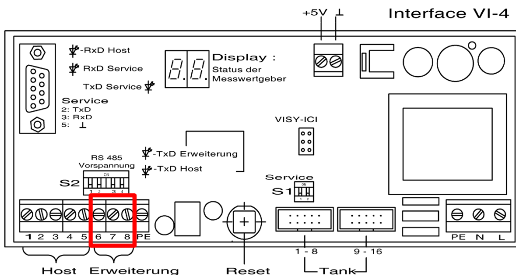
Abbildung 4: Erweiterungsschnittstelle des Interface VI-4
