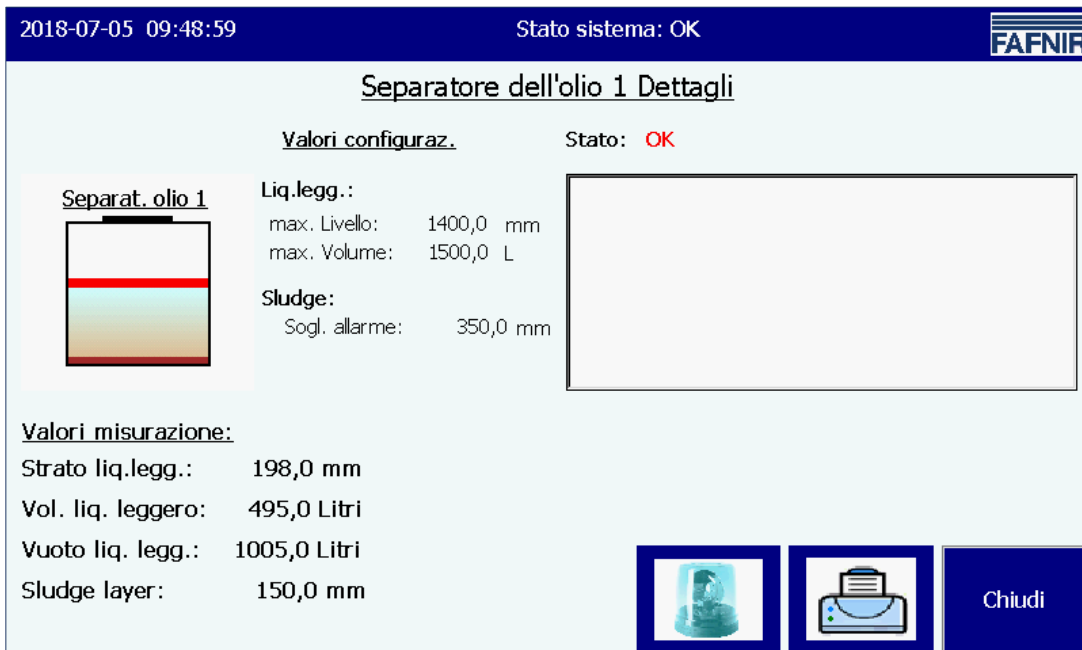
Figura 31: Separatore d'olio basato su VISY-Stick, dettagli
