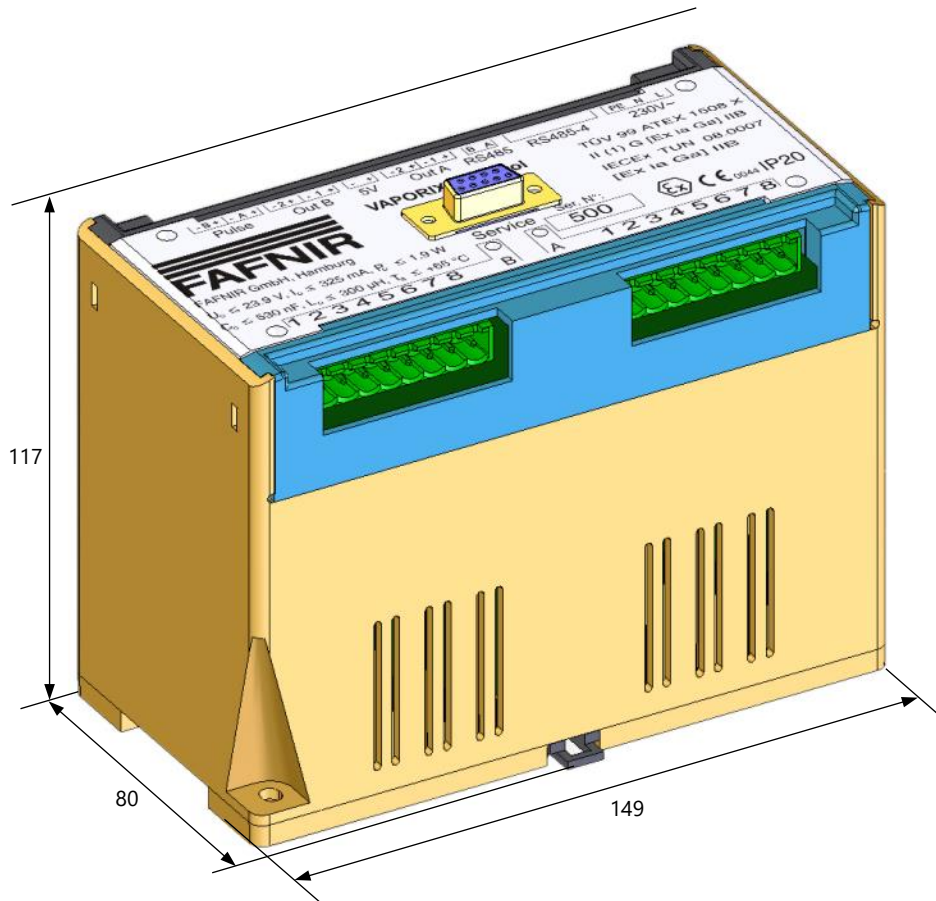
Abbildung 5: Messauswertung VAPORIX-Control
