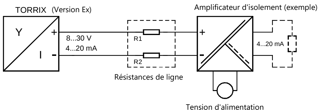
Figure 8 : Schéma de raccordement pour TORRIX Ex
