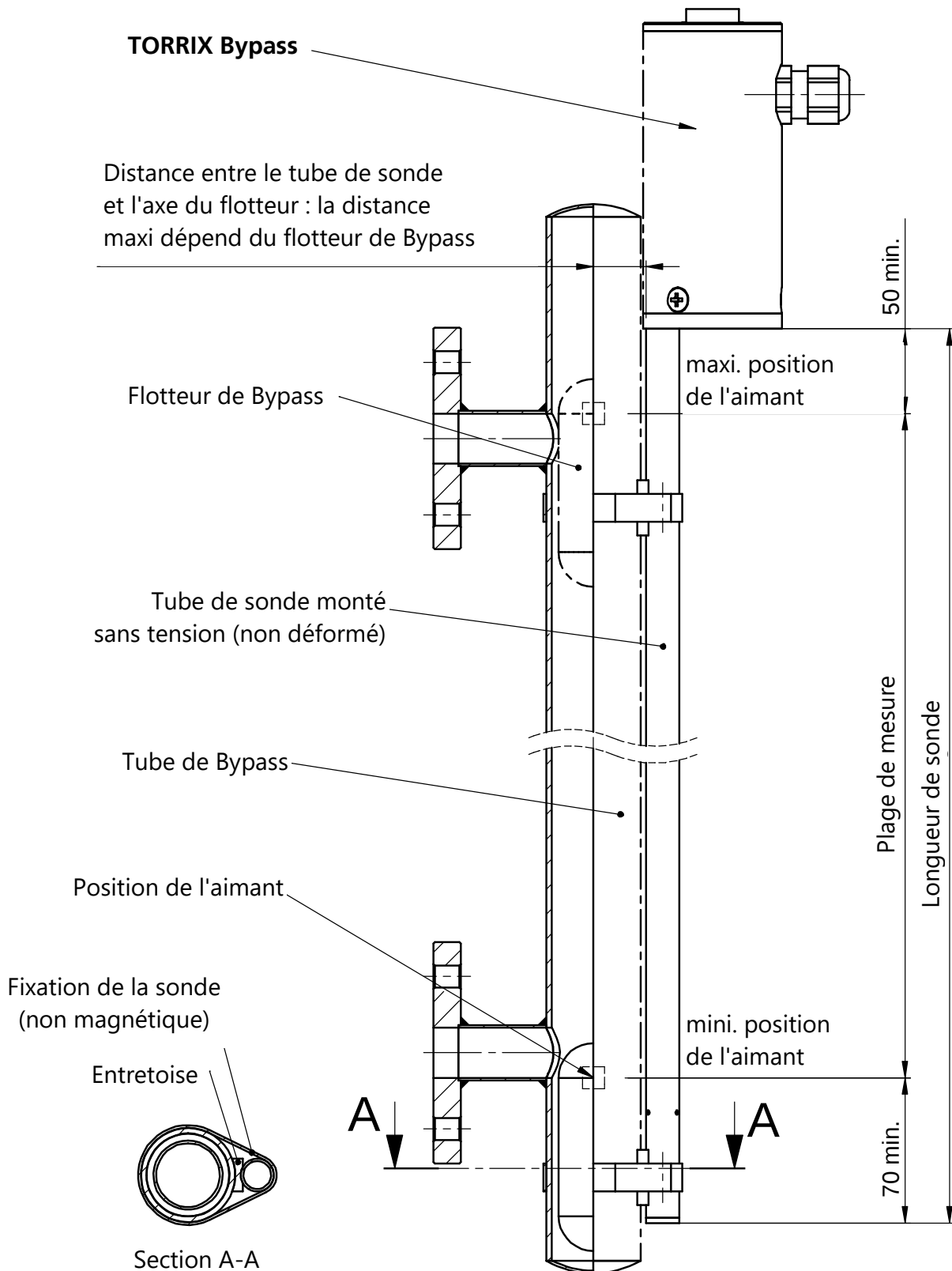
Figure 6 : Montage avec Bypass
