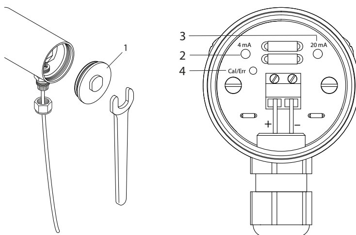
Figure 11 : Ajustage de l'étendue de la plage de mesures
