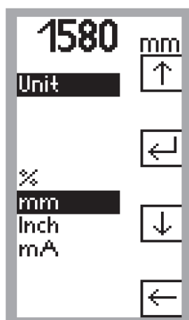
Fig. 13 : affichage « Unit »
