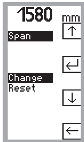
Fig. 16 : affichage « Span »
