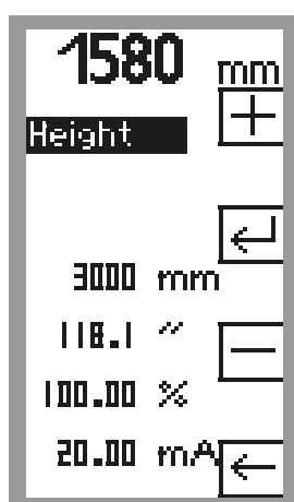
Fig. 14 : affichage « Height »
