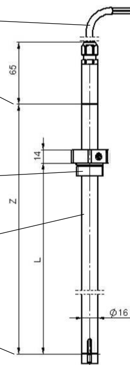
Abb. 5: Standaufnehmer 76 E
