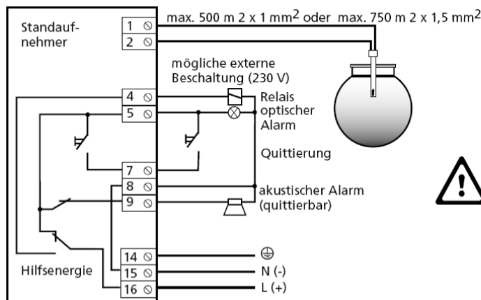
Abb. 31: Anschlussschema NB 220 QS
