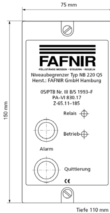
Abb. 21: Maßblatt NB 220 QS
