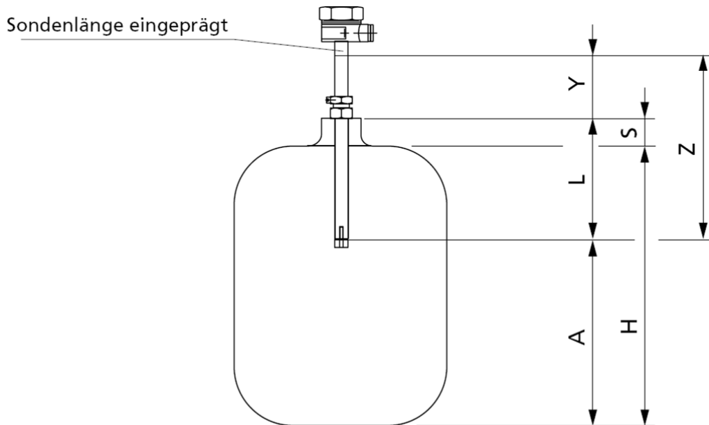
Abb. 33: Einstellmaße
