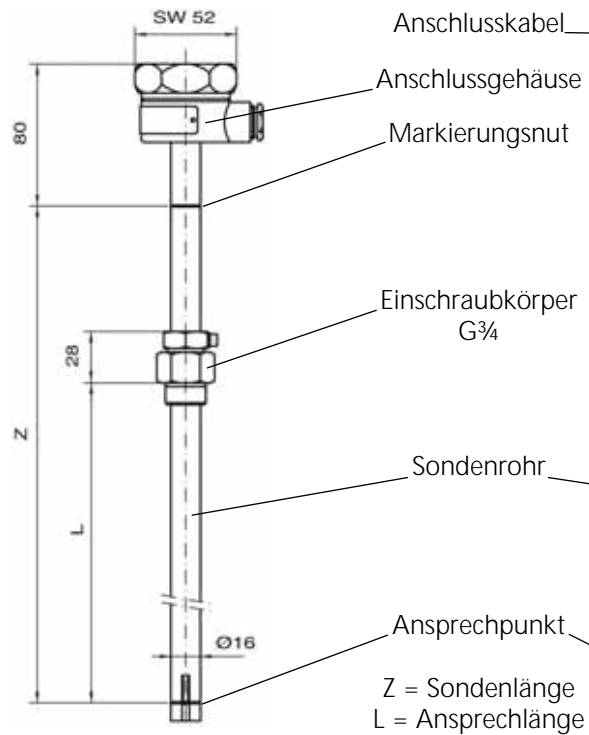
Abb. 4: Standaufnehmer 76 C
