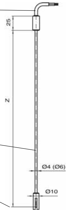
Abb. 5: Standaufnehmer 76 E
