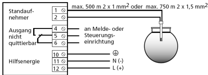
Abb. 30: Anschlussschema NB 220 H
