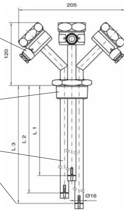
Abb. 11: Standaufnehmer 76 TRIO 1
