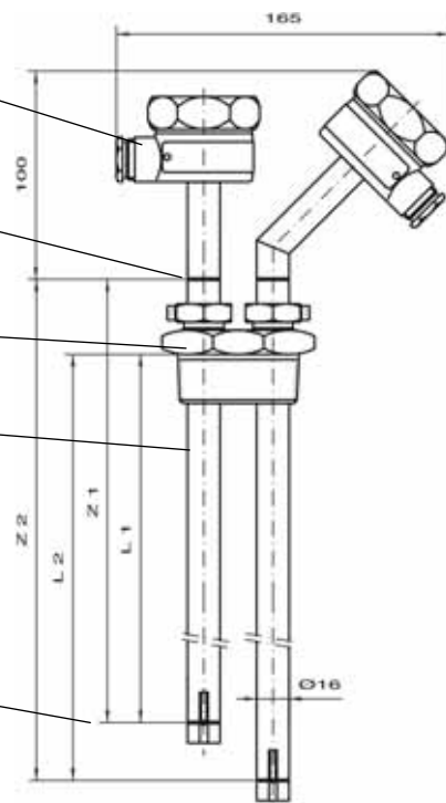
Abb. 9: Standaufnehmer 76 DUO 2
