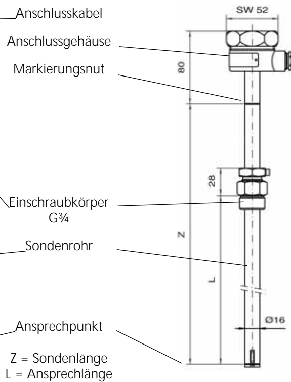
Abb. 9: Standaufnehmer 76 DUO 2
