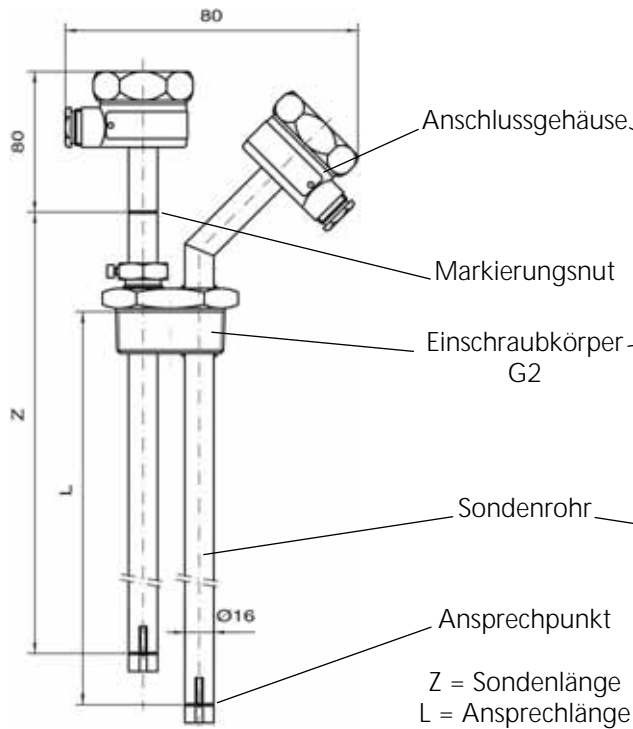
Abb. 12: Standaufnehmer 76 A TRIO 3
