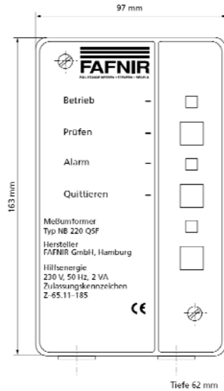
Abb. 22: Maßblatt NB 220 QSF
