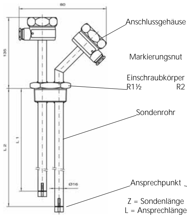
Abb. 8: Standaufnehmer 76 A DUO 1
