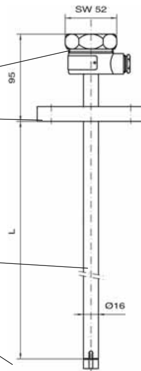
Abb. 13: Standaufnehmer 76 A F
