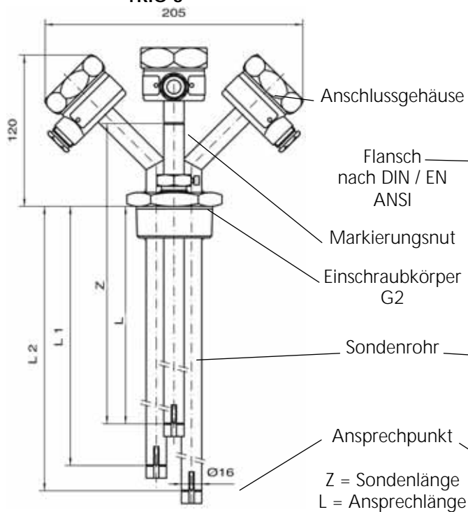
Abb. 12: Standaufnehmer 76 A TRIO 3
