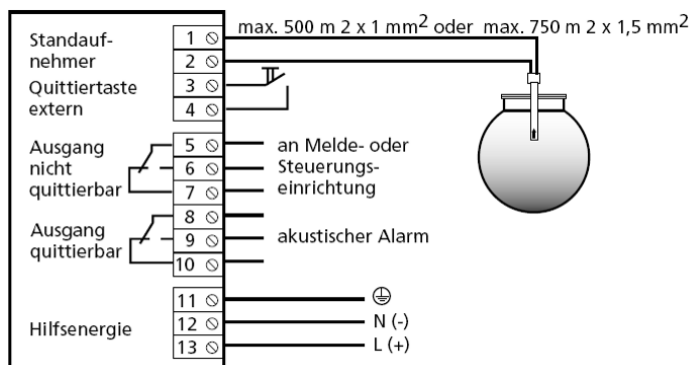
Abb. 32: Anschlussschema NB 220 QSF
