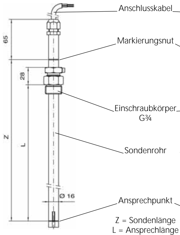
Abb. 4: Standaufnehmer 76 C
